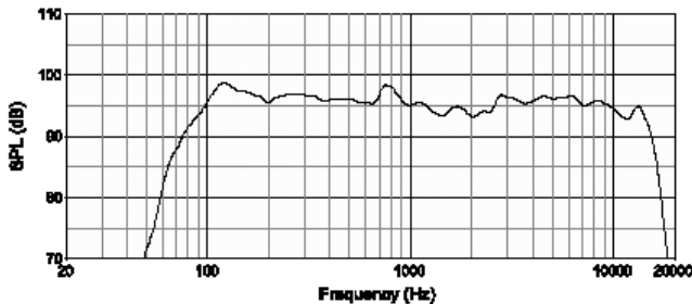
Courbe de réponse dans un demi-espace
