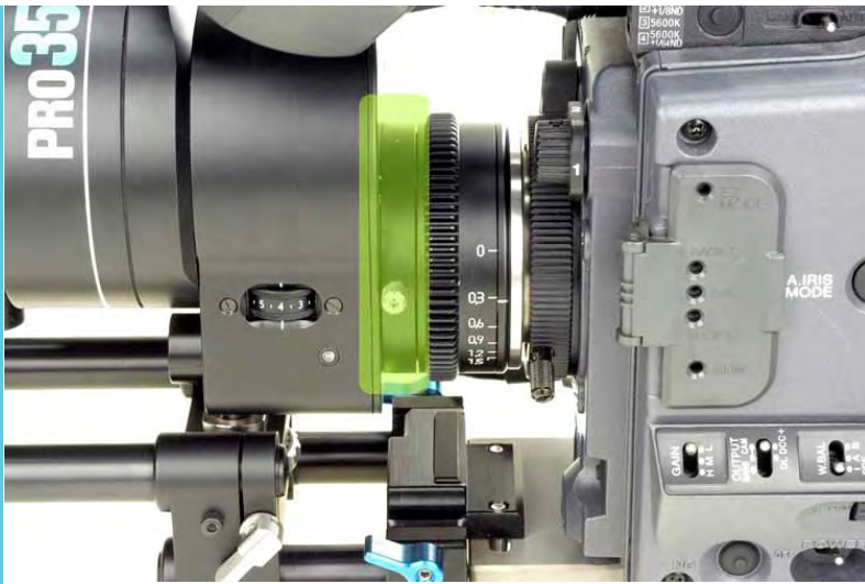
Bague de mise au point arrière ou back-focus
