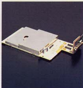
BKU-701 Carte d'interfaçage ordinateur RS 232 C
